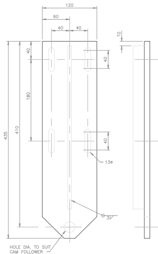
DETAIL -- ITEM 21
